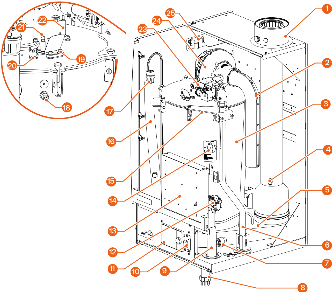
Fig. 2. Composants de la chaudière
