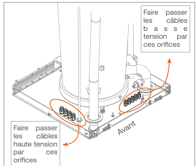
Fig. 15. Cheminement des câbles électriques - N 60 à 120 WH
