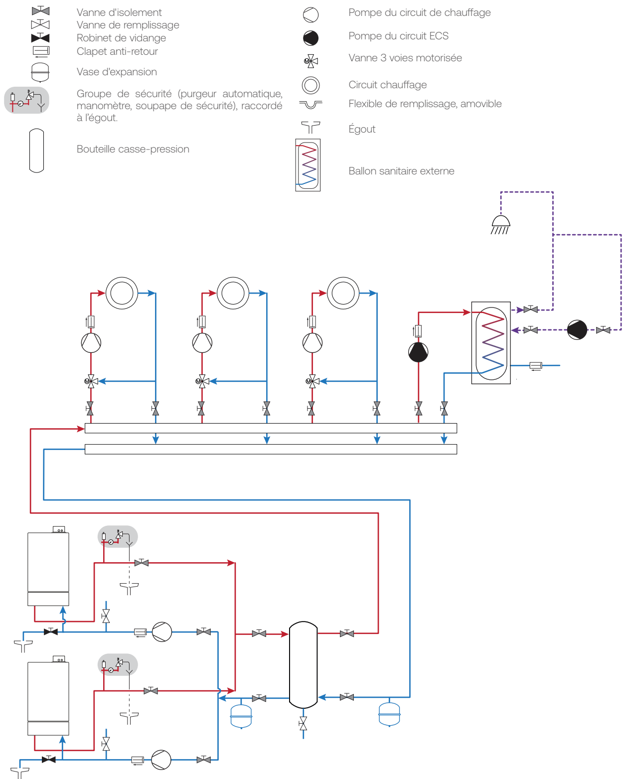
Fig. 13. Chaudières en cascade, avec ballon sanitaire externe et bouteille casse-pression
