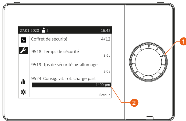
Fig. 28. Réglage du régime du ventilateur - écran type
