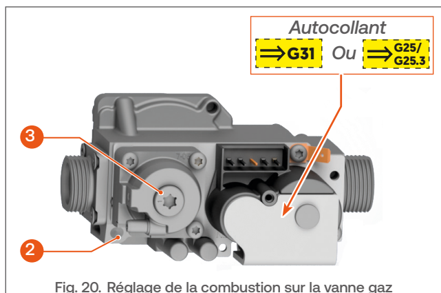
Fig. 20. Réglage de la combustion sur la vanne gaz
