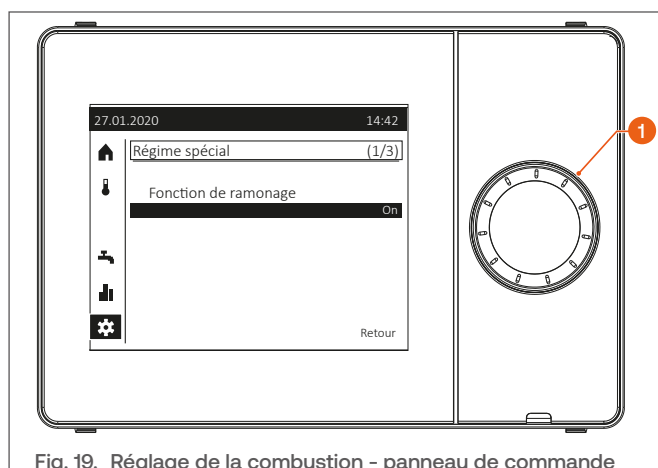
Fig. 19. Réglage de la combustion - panneau de commande
