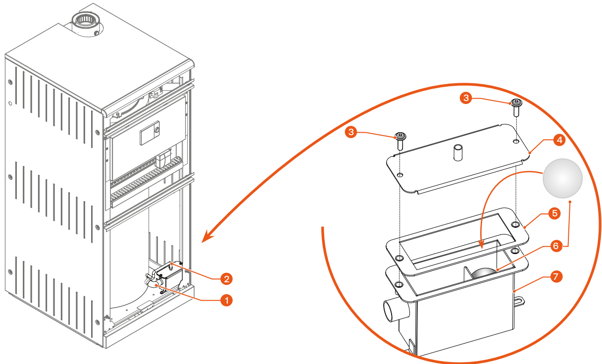
Fig. 22. Nettoyer le conduit et le collecteur de condensats.
