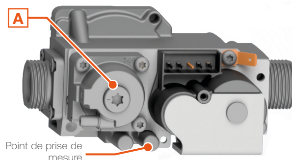
Fig. 11. Vanne gaz
