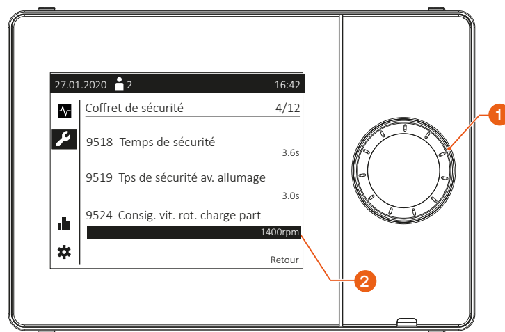
Fig. 18. Réglage du régime du ventilateur - écran type
