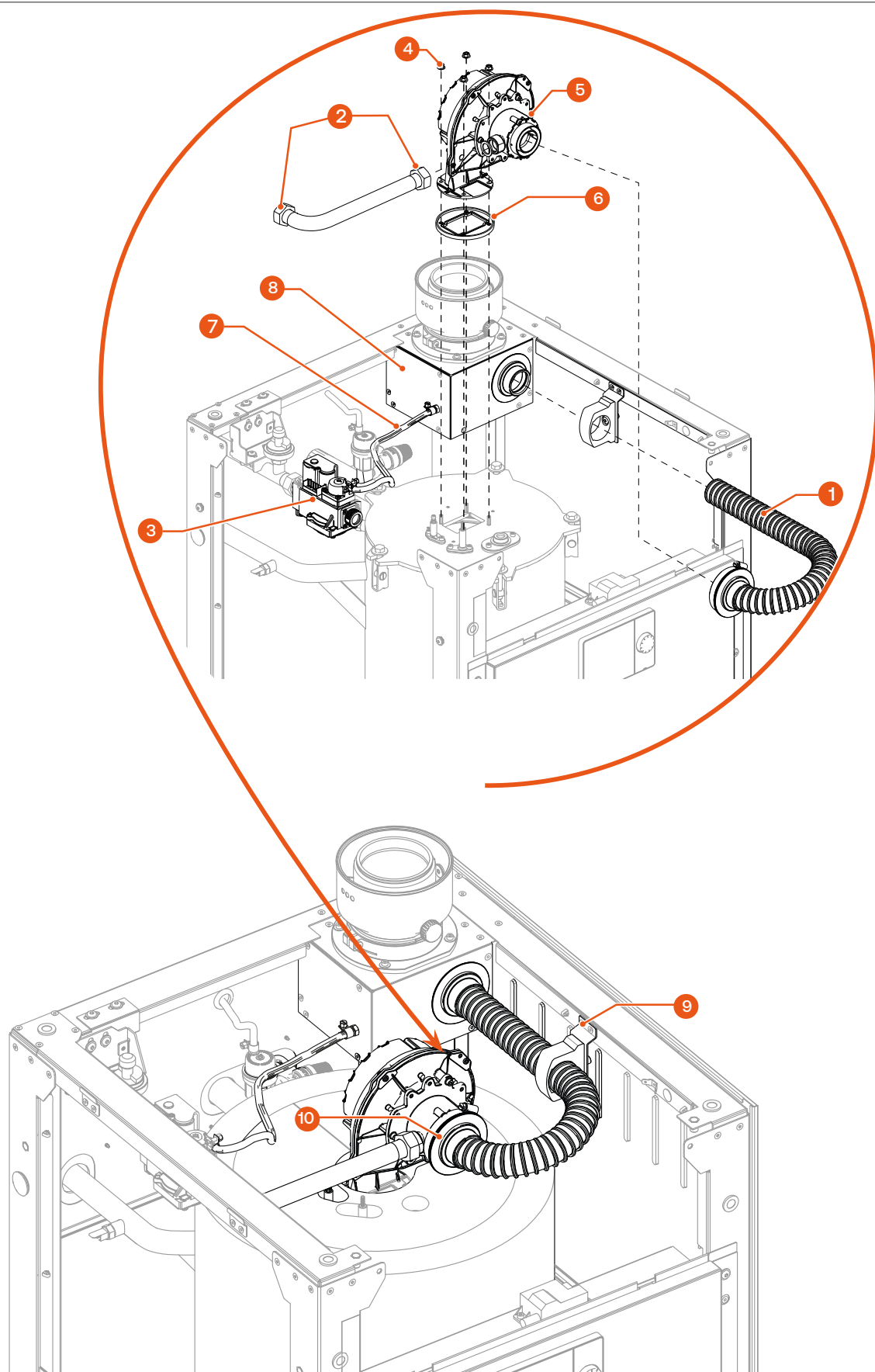
Fig. 24. Démontez et installez l'ensemble ventilateur et dispositif de mélange air-gaz
