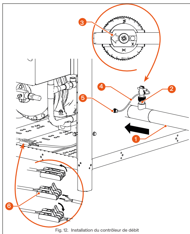
Fig. 12. Installation du contrôleur de débit
