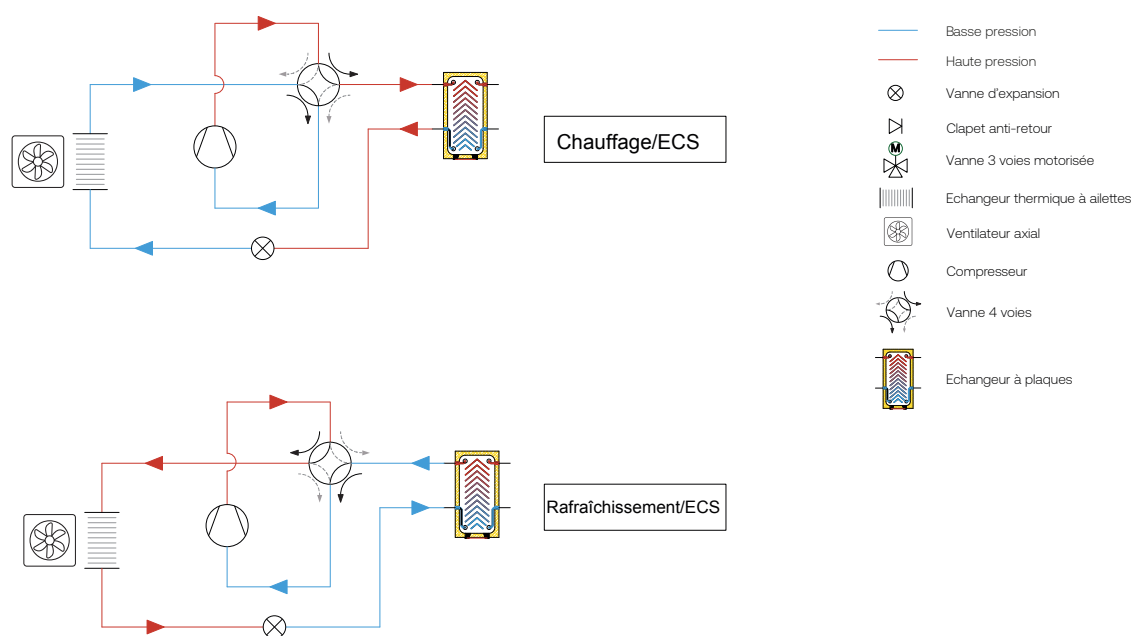
Fig. 17. Schéma de principe du rafraîchissement - système 2 tubes
