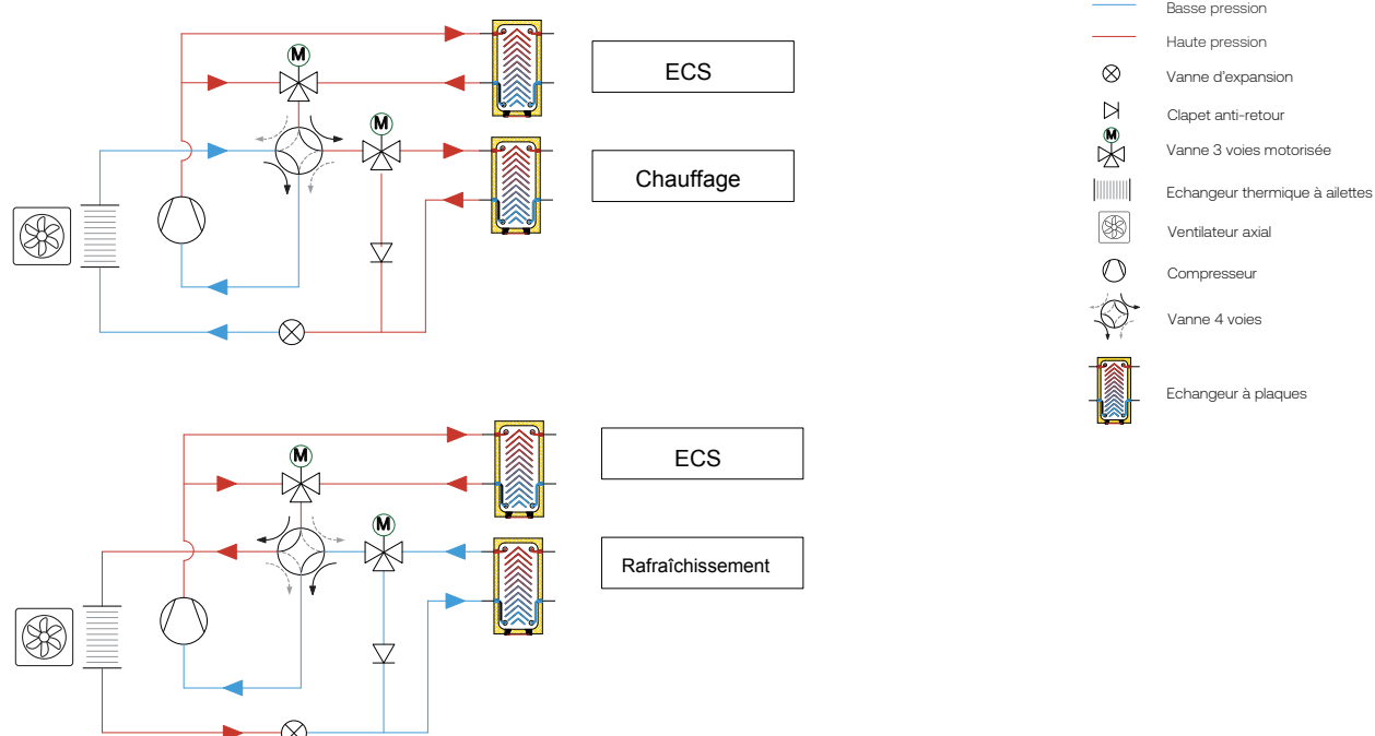
Fig. 18. Schéma de principe du rafraîchissement - système 4 tubes
